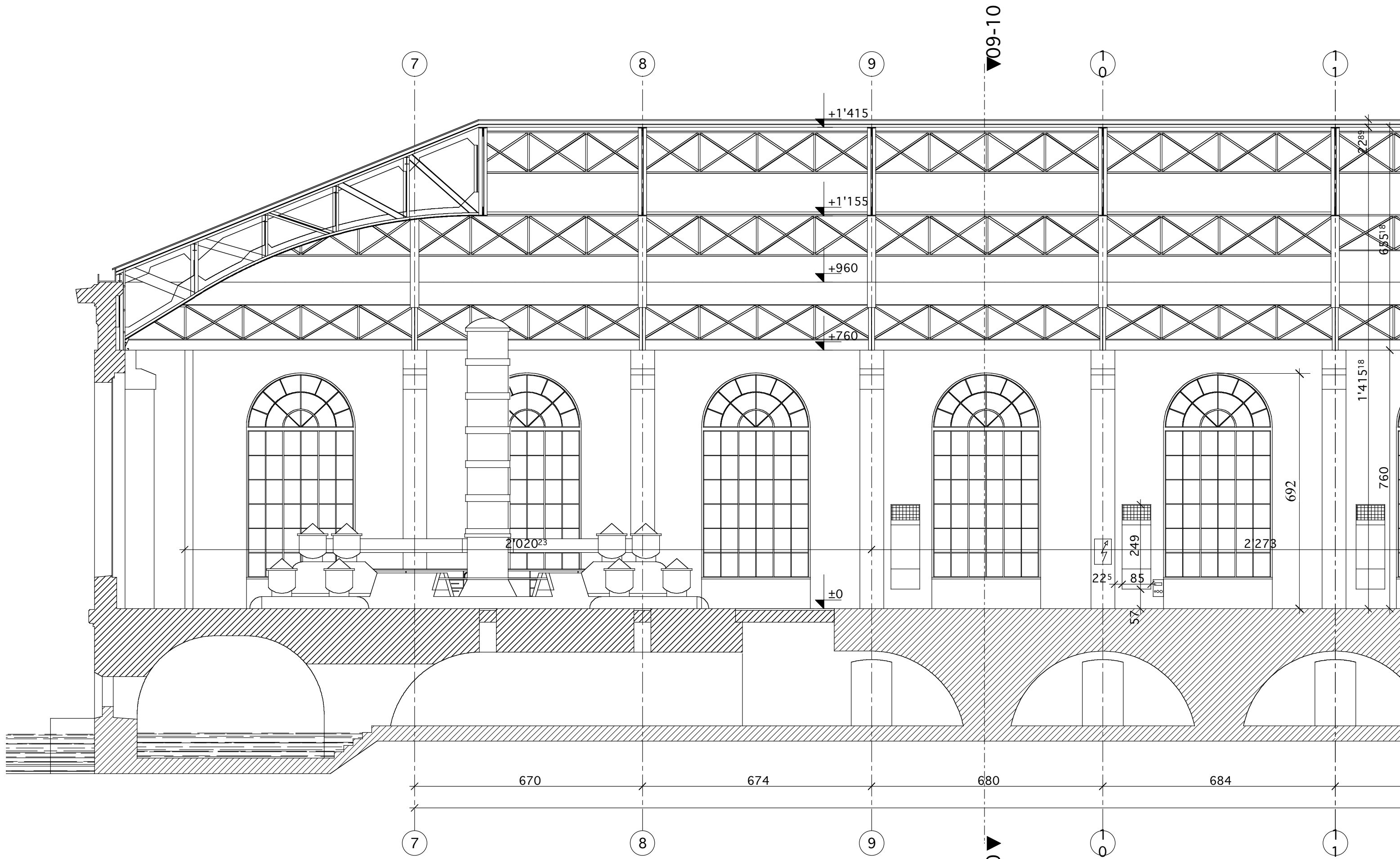
COUPE LONGITUDINALE A-A PARTIE 1/2 ESPACE POLYVALENT BFM
