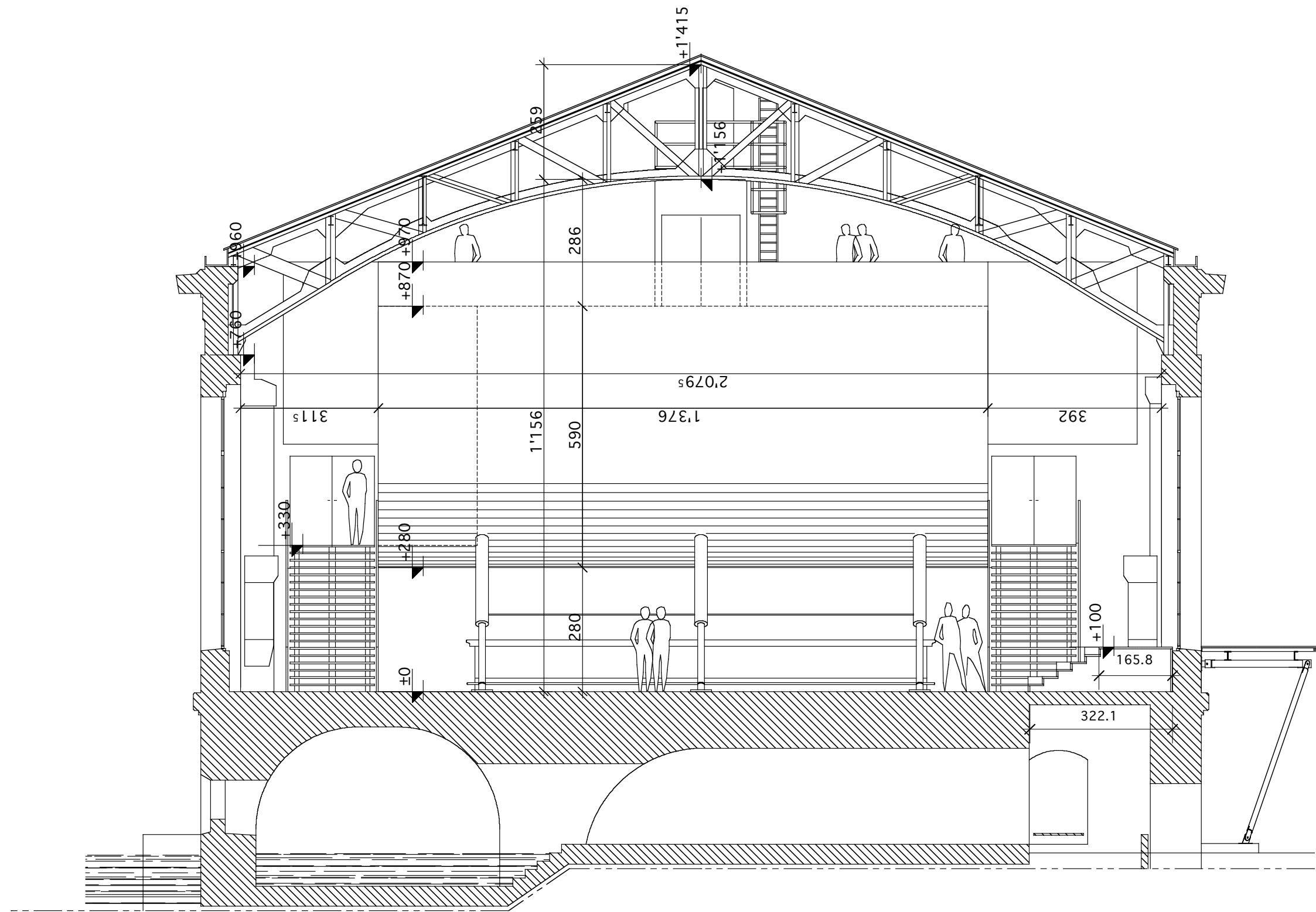
COUPE TRANSVERSALE AXES 09-10
