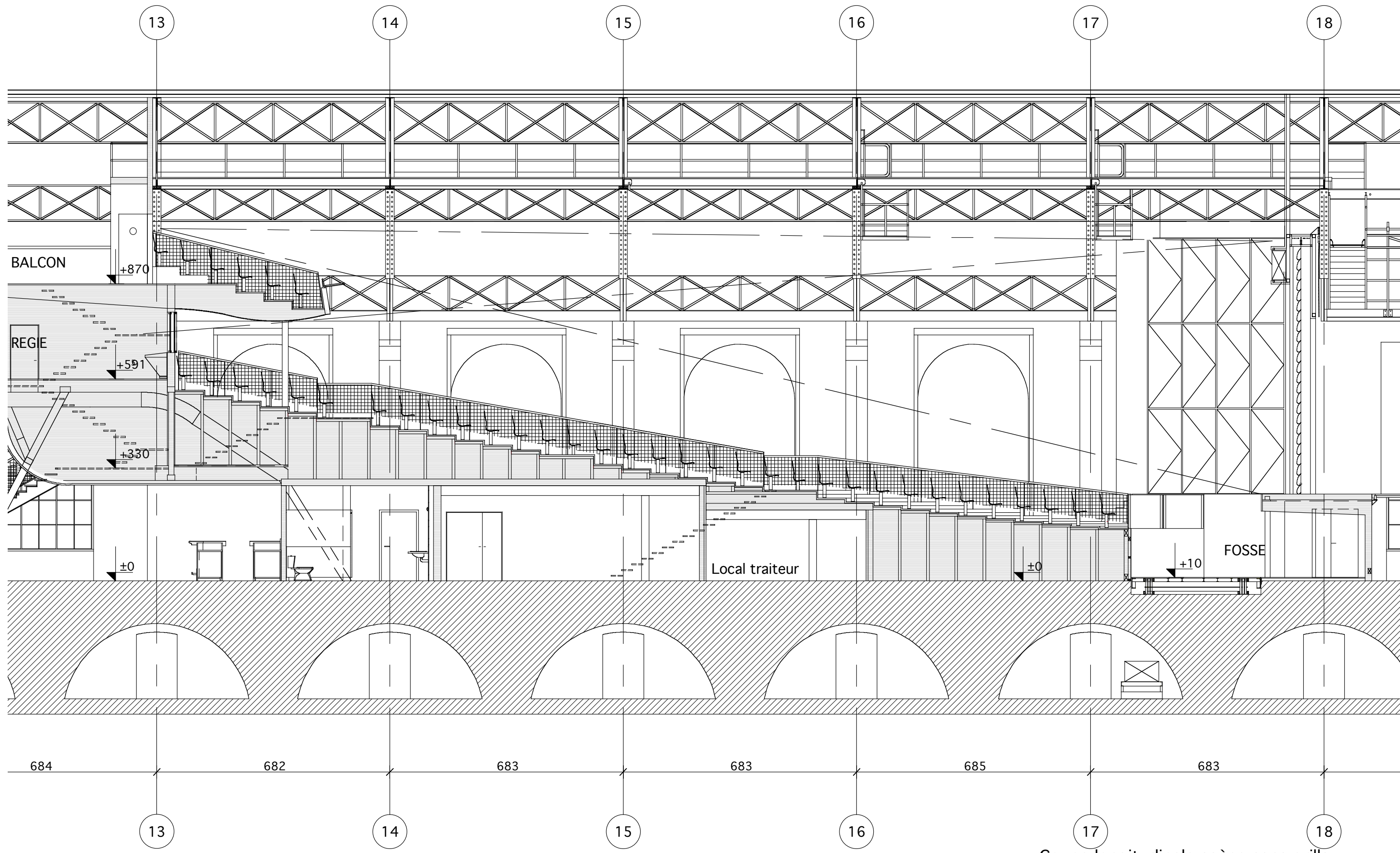
Coupe longitudinale scène sans grills Régie - Fosse BFM 1:100
