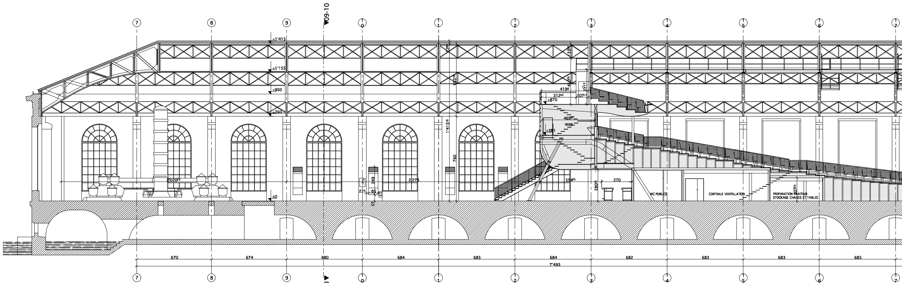
COUPE LONGITUDINALE A-A
